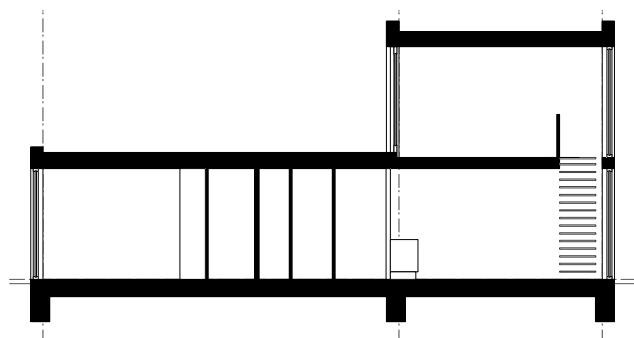
doorsnede A-A
