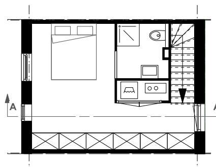
plattegrond verdieping 2
