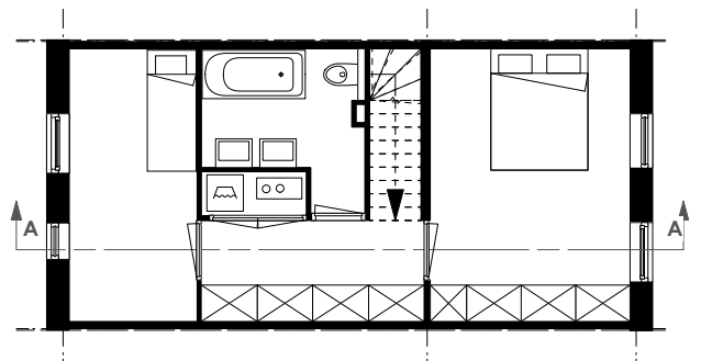
plattegrond verdieping 2
