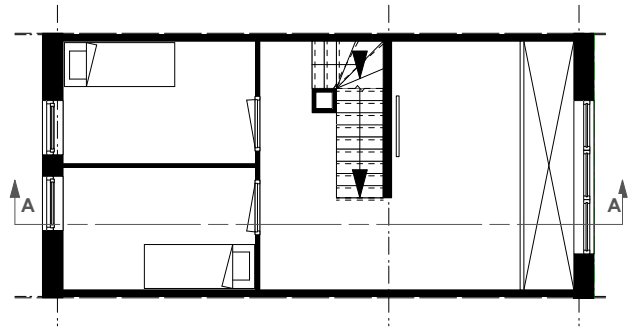
plattegrond verdieping 1
