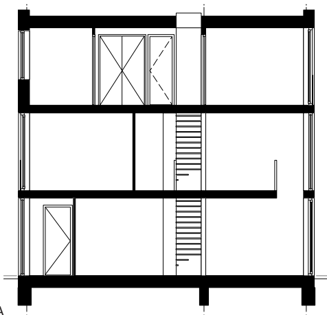
doorsnede A-A
