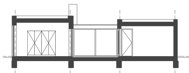
doorsnede A-A
