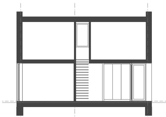
doorsnede A-A
