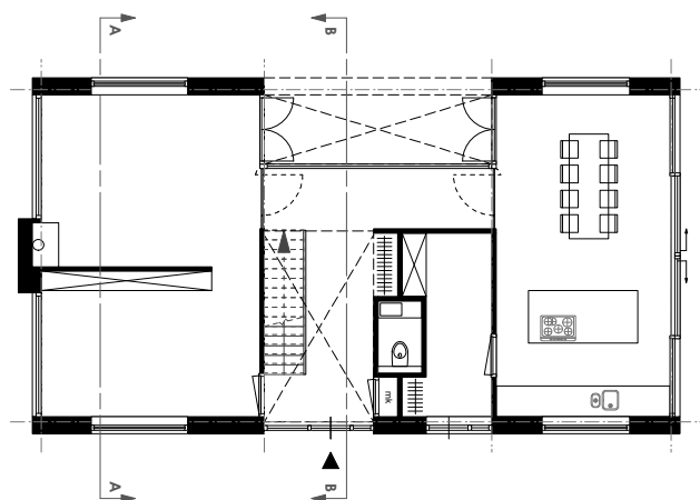
plattegrond begane grond
