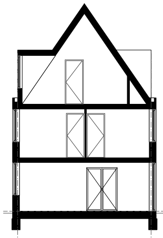
doorsnede A-A
