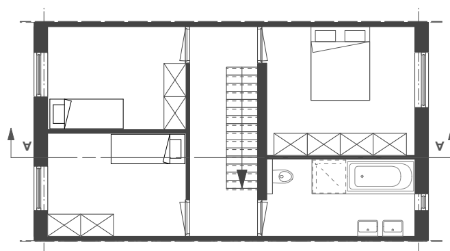
plattegrond verdieping 2
