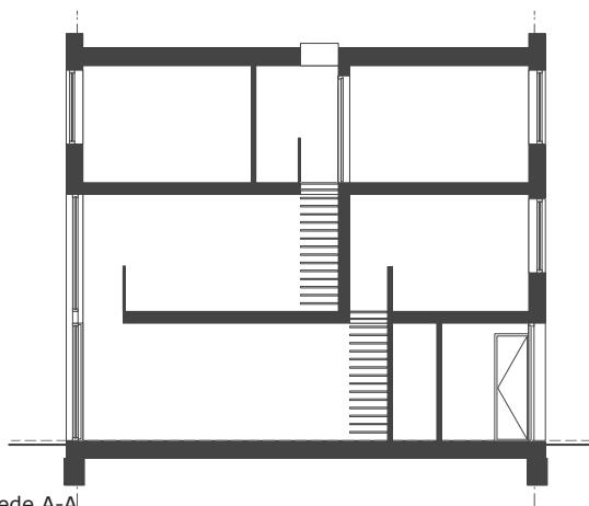
doorsnede A-A
