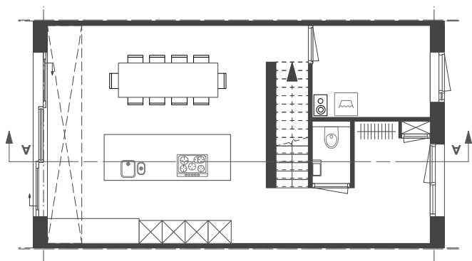
plattegrond begane grond
