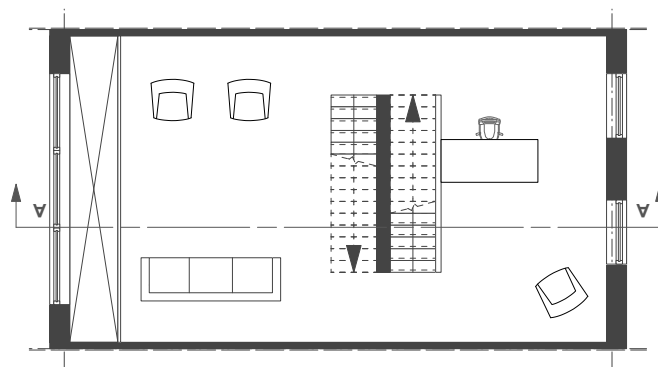
plattegrond verdieping 1
